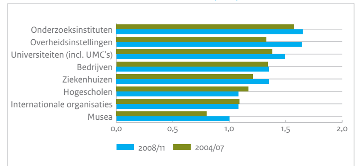
Figuur 10.11 Citatie-impact
