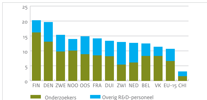
Figuur 10.4 R&D-personeel
